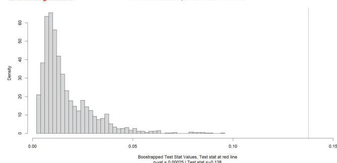
Figure 4. Test quadratique de Wasserstein entre la distribution des déciles de la Belgique et celle de l'Autriche
