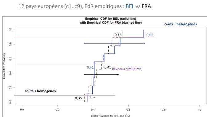
Figure 7. Comparaison graphique entre les fonctions de répartition des déciles estimés de coûts unitaires, Belgique versus France
