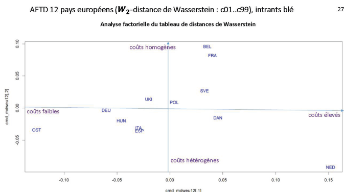
Figure 8. AFTD des distributions de centiles estimés de 12 pays européens
