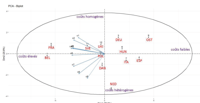
Figure 2. Biplot des distributions de déciles estimés de 12 pays européens
