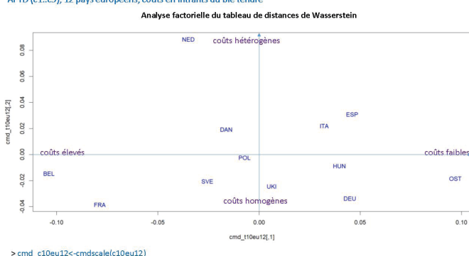
Figure 1. AFTD des distributions de déciles estimés de 12 pays européens
