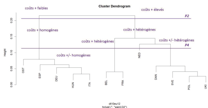
Figure 3. Dendrogramme de la CAH sur tableau des distances de Wasserstein entre les distributions de déciles estimés pour 12 pays européens
