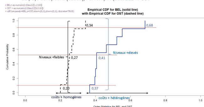
Figure 5. Comparaison graphique entre la distribution des déciles de la Belgique et celle de l'Autriche
