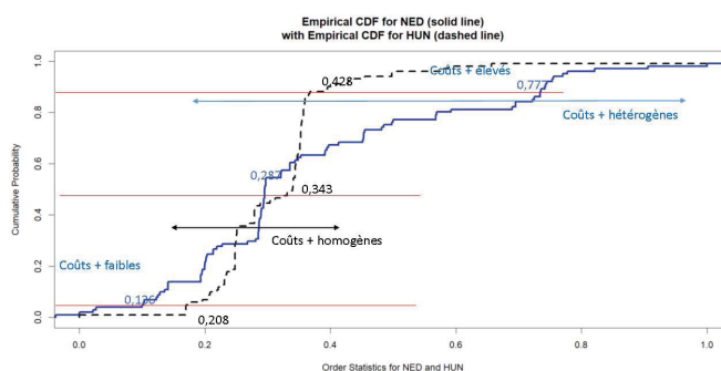
Figure 10. Comparaison graphique entre les distributions quantiles des Pays-Bas et de la Hongrie
