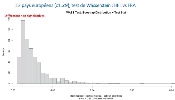
Figure 6. Test quadratique de Wasserstein entre la distribution des déciles de la Belgique et celle de la France
