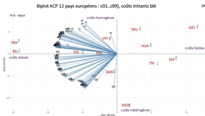
Figure 9. Biplot de l'ACP du tableau des centiles estimés de 12 pays européens
